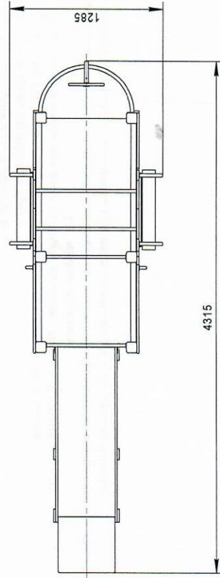
Рисунок 1 - Общий вид изделия
